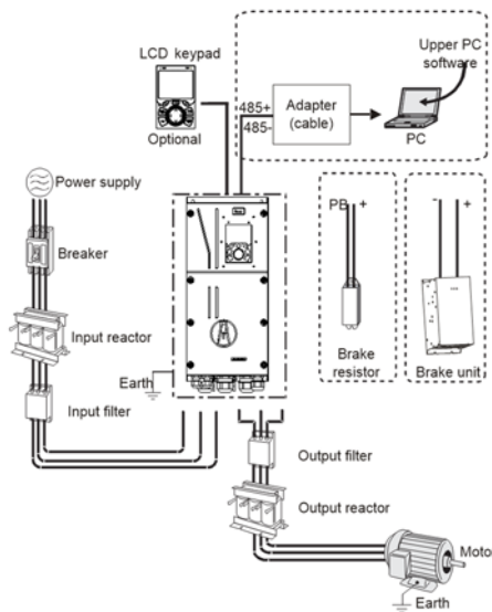
Figur 1-2 ST600SP ledningsføring
