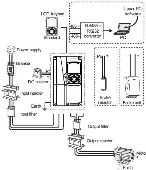
Figur 1-1 ST600 ledningsføring
