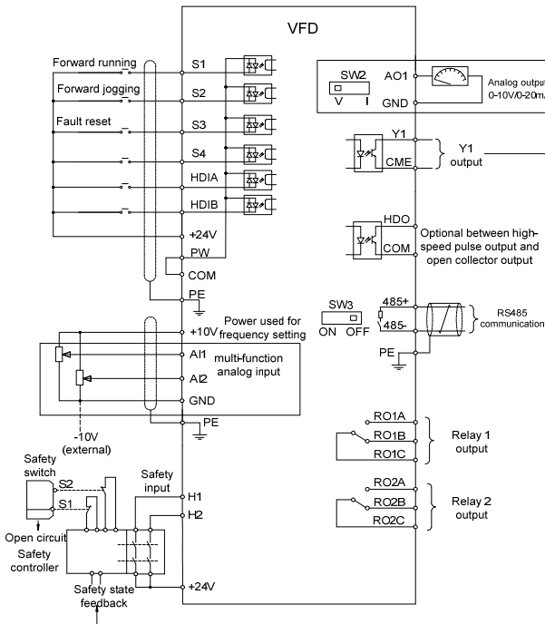
Figur 2-1 Generel ledningsføring
